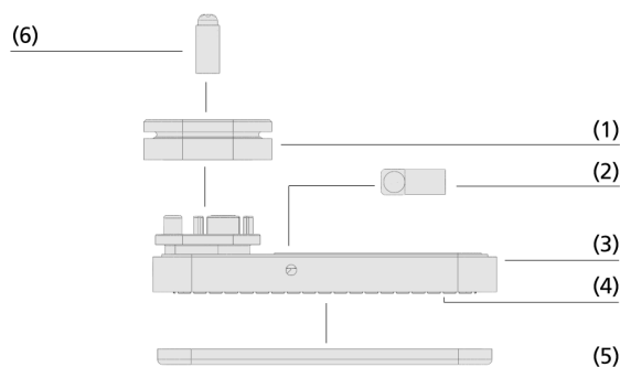
Design del sistema Blocchi di aspirazione VCBL-G-K1
